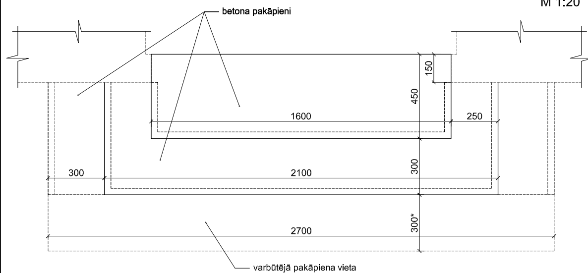
KĀPŅU VIRSSKATS M 1:20
