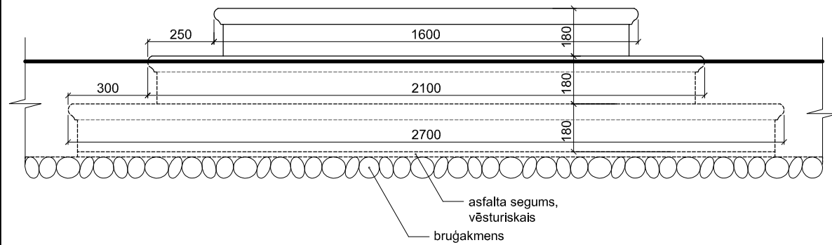
KĀPŅU VIRSSKATS M 1:20
