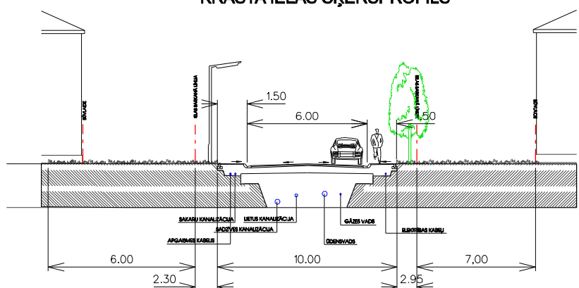
ŠKĒLUMS 2-2 KRASTA IELAS ŠKĒRSPROFILS
