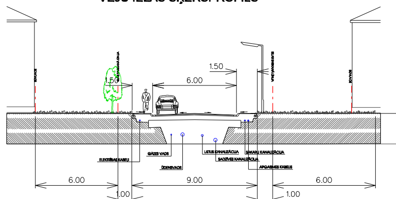
ŠKĒLUMS 1-1 VĒJU IELAS ŠKĒRSPROFILS
