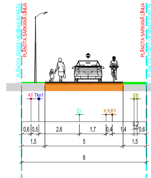
GRIEZUMS 4 - 4
