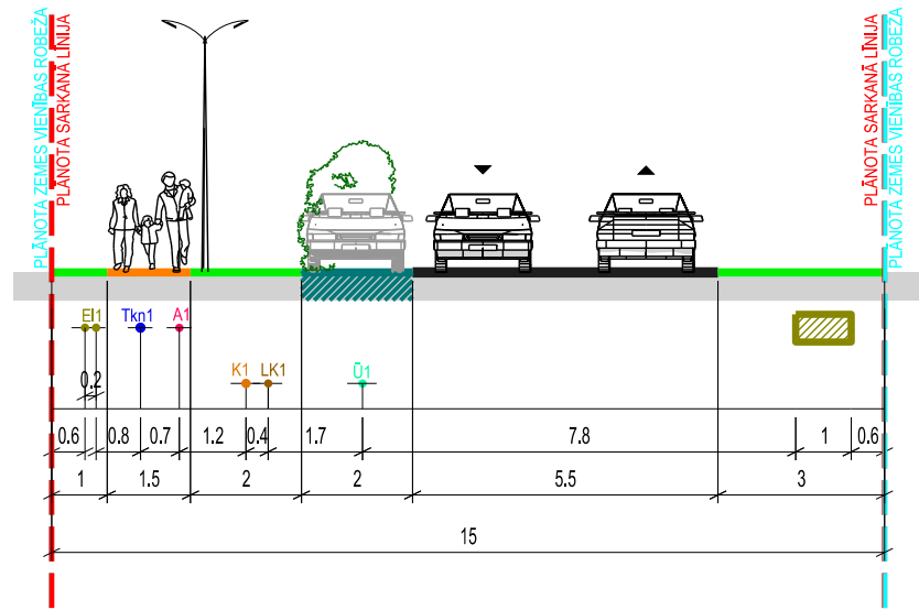
PLĀNOTĀS IELAS A ŠĶĒRSPROFILS GRIEZUMS 1 - 1
