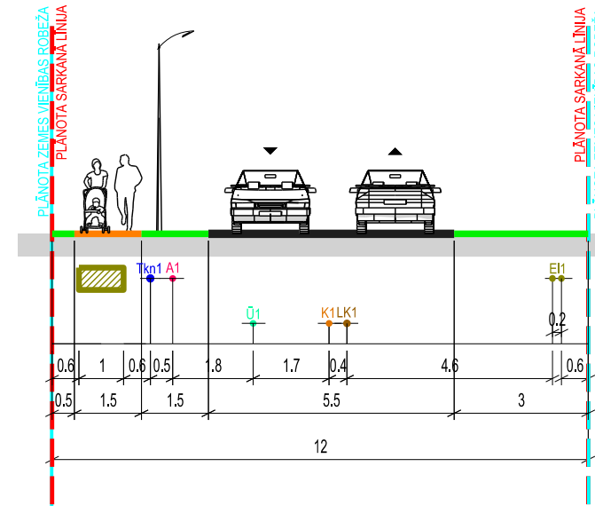
PLĀNOTĀS IELAS B ŠĶĒRSPROFILS GRIEZUMS 3 - 3
