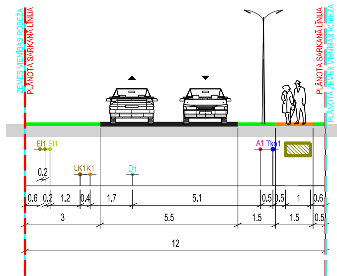
PLĀNOTO IELU B UN C ŠĶĒRSPROFILS GRIEZUMS 2 - 2
